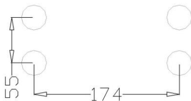
Rozstaw fundamentów
